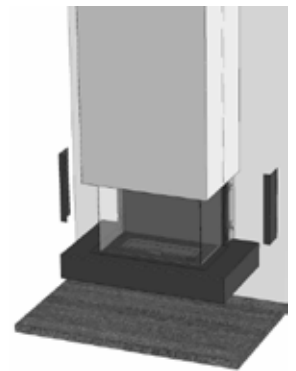
INSTALLATION DES PANNEAUX LATÉRAUX
