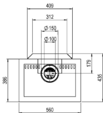
MODULE SIMPLE : H 200 mm
